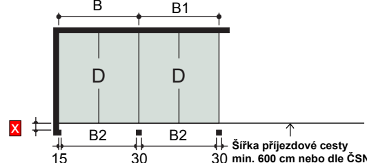
dvojaráž (4 vozidla)
