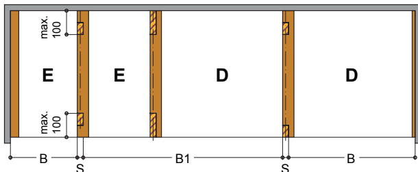
Jednoduché zařízení
