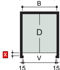
dvojaráž (4 vozidla)
